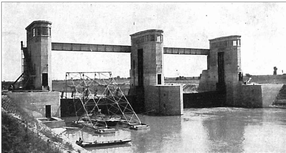
A Horthy István duzzasztómű az alvíz felől nézve. A baloldali nyílásközben egy úszódaru látható
