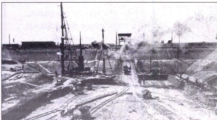
1938. június 2. Az alappödröt és az alaplemezt körülzáró vasszádfal leverése
